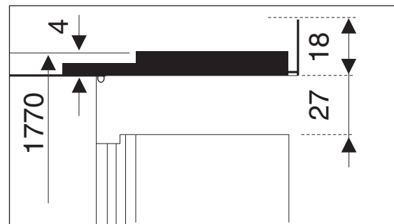
Zijaanzicht bovenzijde
