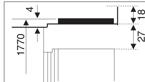
Zijaanzicht bovenzijde
