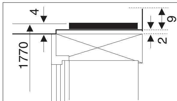
Zijaanzicht bovenzijde
