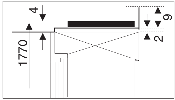
Zijaanzicht bovenzijde
