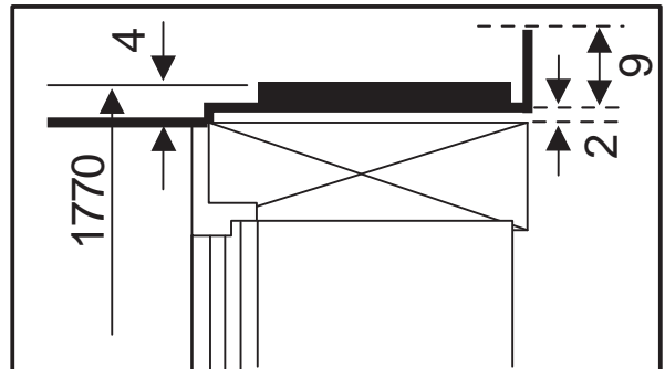
Zijaanzicht bovenzijde/side view top
