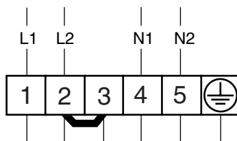
fig. 18: Aansluitschema
