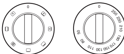
fig. 10: Functieknop + thermostaatknop
