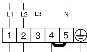
fig. 17: Aansluitschema
