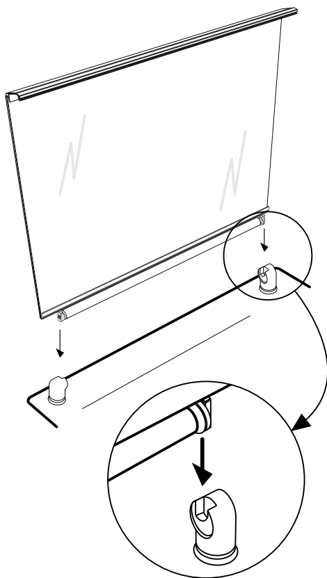
fig. 18: Plaatsen glazen sierdeksel
