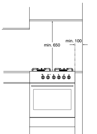
fig. 19: Opstelling
