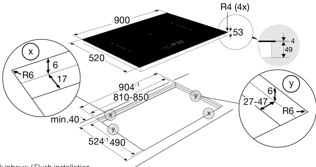
Vlak inbouw / Flush installation
