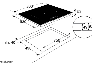
Opbouw / Top installation
