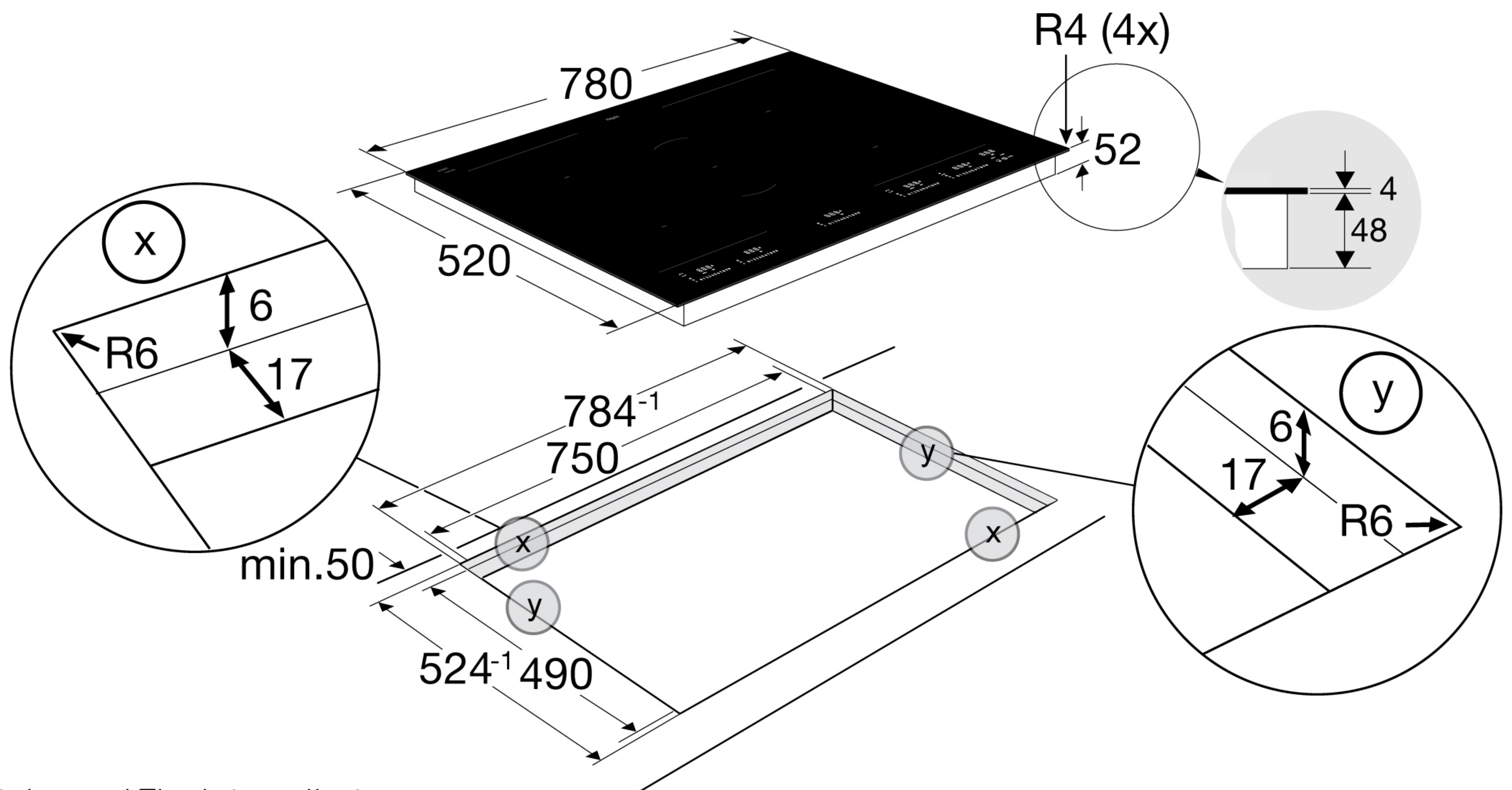
Vlak inbouw / Flush installation
