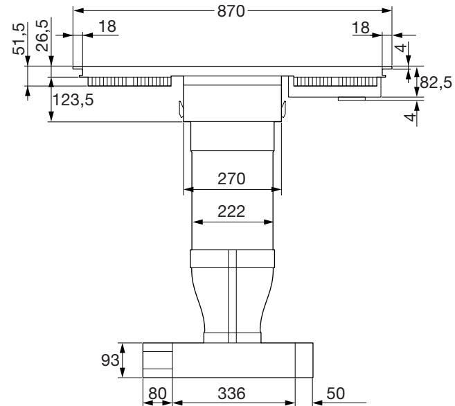
Vooraanzicht
