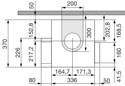
Wandopstelling
