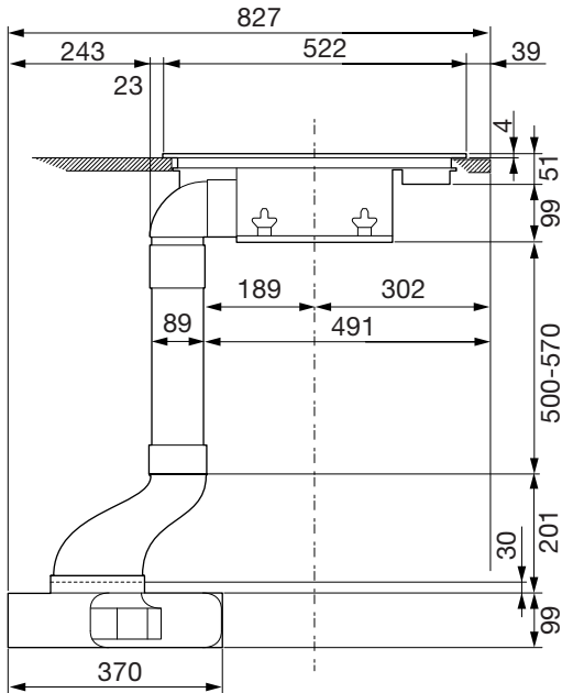
Eilandopstelling
