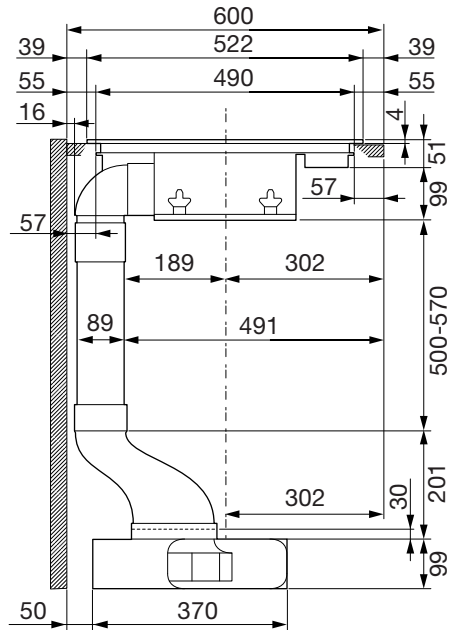
Wandopstelling
