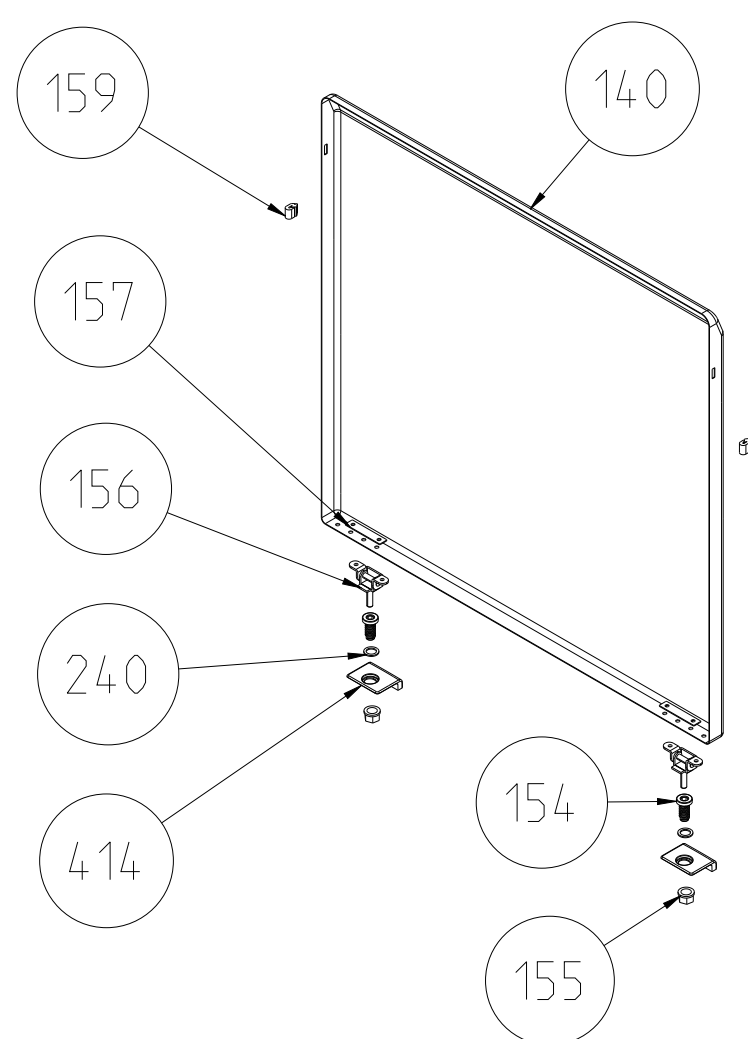
METAL LID OPTIONAL (POSITION NO 153)
