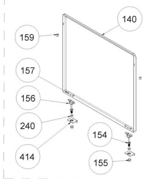
METAL LID OPTIONAL (POSITION NO 153)
