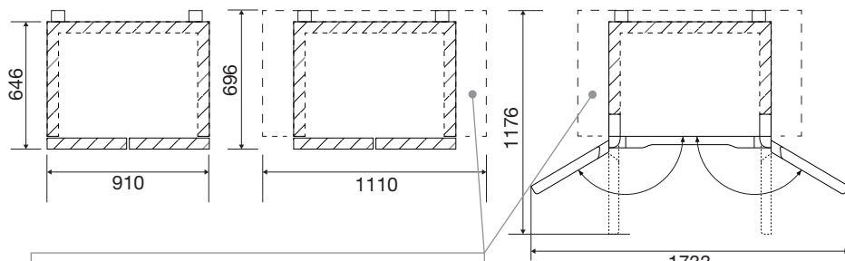
Totale afmetingen
