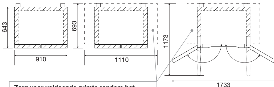
Totale afmetingen
