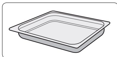
5 Groot stoomovenbakblik zonder gaten, 40 mm diep, Gastro-Norm-maat GN 2/3 (geschikt voor het opvangen van condens tijdens het stomen, niveau 2, 3, 4 en 5)
