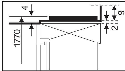
Zijaanzicht bovenzijde/side view top
