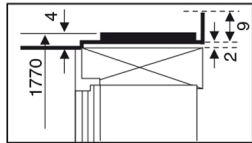
Zijaanzicht bovenzijde
