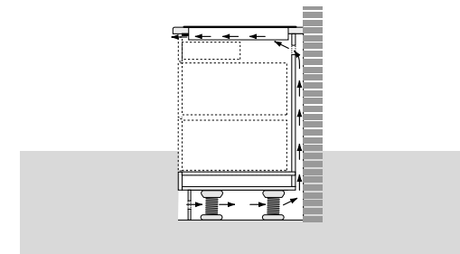
Luchtcirculatie onder de inductiekookplaat.
